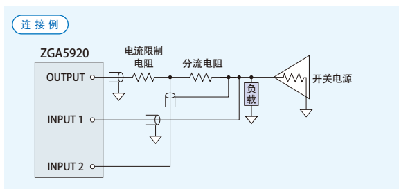
每个负载的开关电源输出阻抗▶
