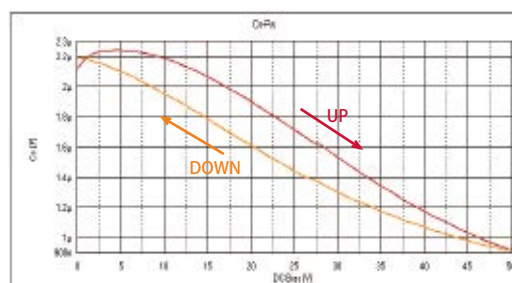
▲根据 DC 偏压扫描方向测量电容的磁滞
