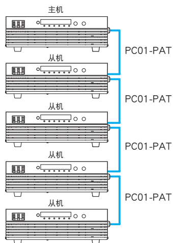
并联运行电缆 PC01-PAT
